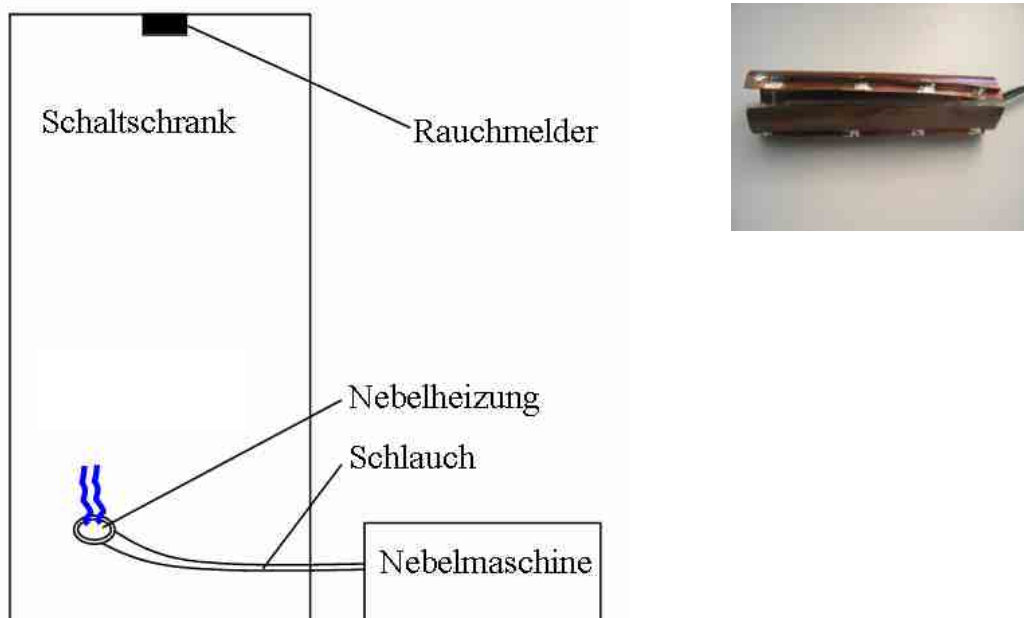
Abbildung 2: Testaufbau für Technikraumtest / Nebelheizung für Schlauch
