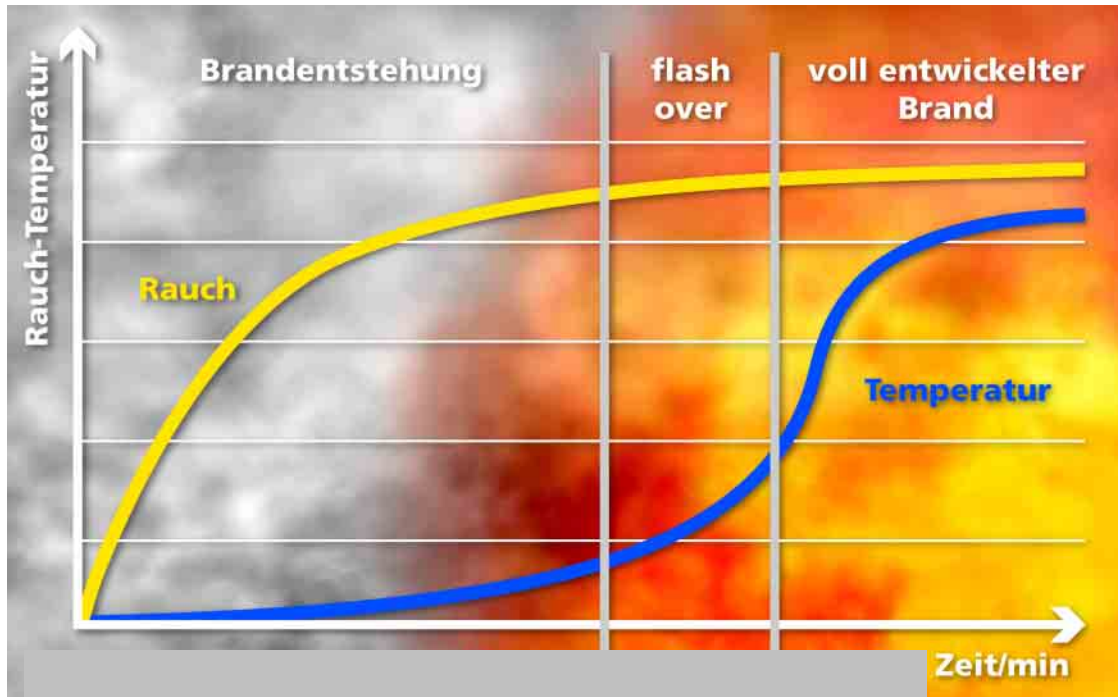
Abbildung 1: Prinzipielle Rauch- und Temperaturentwicklung über den Brandverlauf (Entwicklung ausgehend von einem Schmel- bis zum Flammenbrand)
